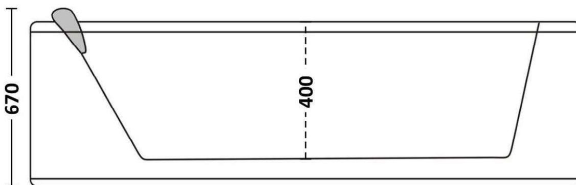
Схема 2. Габаритні розміри Iris TLP-679, мм
