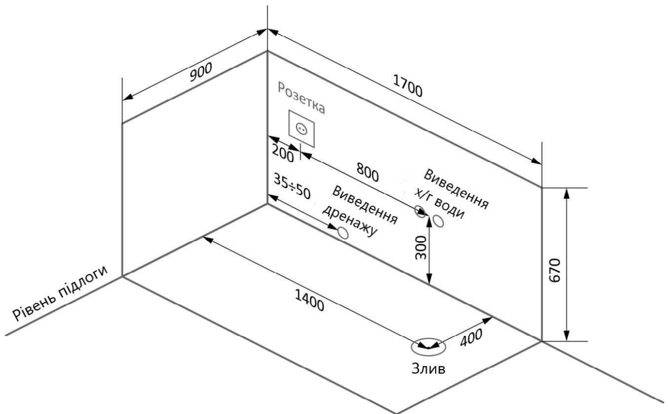
Схема 3. Підведення комунікацій, мм
